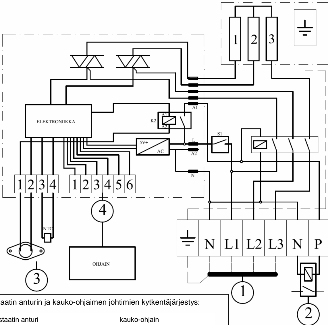
Kytkentäkaavio
